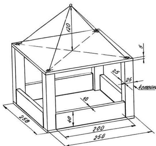
Рисунок 2. Подвесная кормушка
